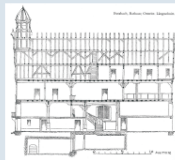
Aufmaße des Rathauses nach Heinrich Winter, Das Bürgerhaus in Oberhessen (Tübingen 1965).
